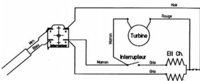
Schema de Cablage 1505 7BB
