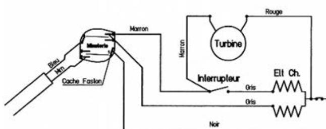
Schema de Cablage 1505 7MB
